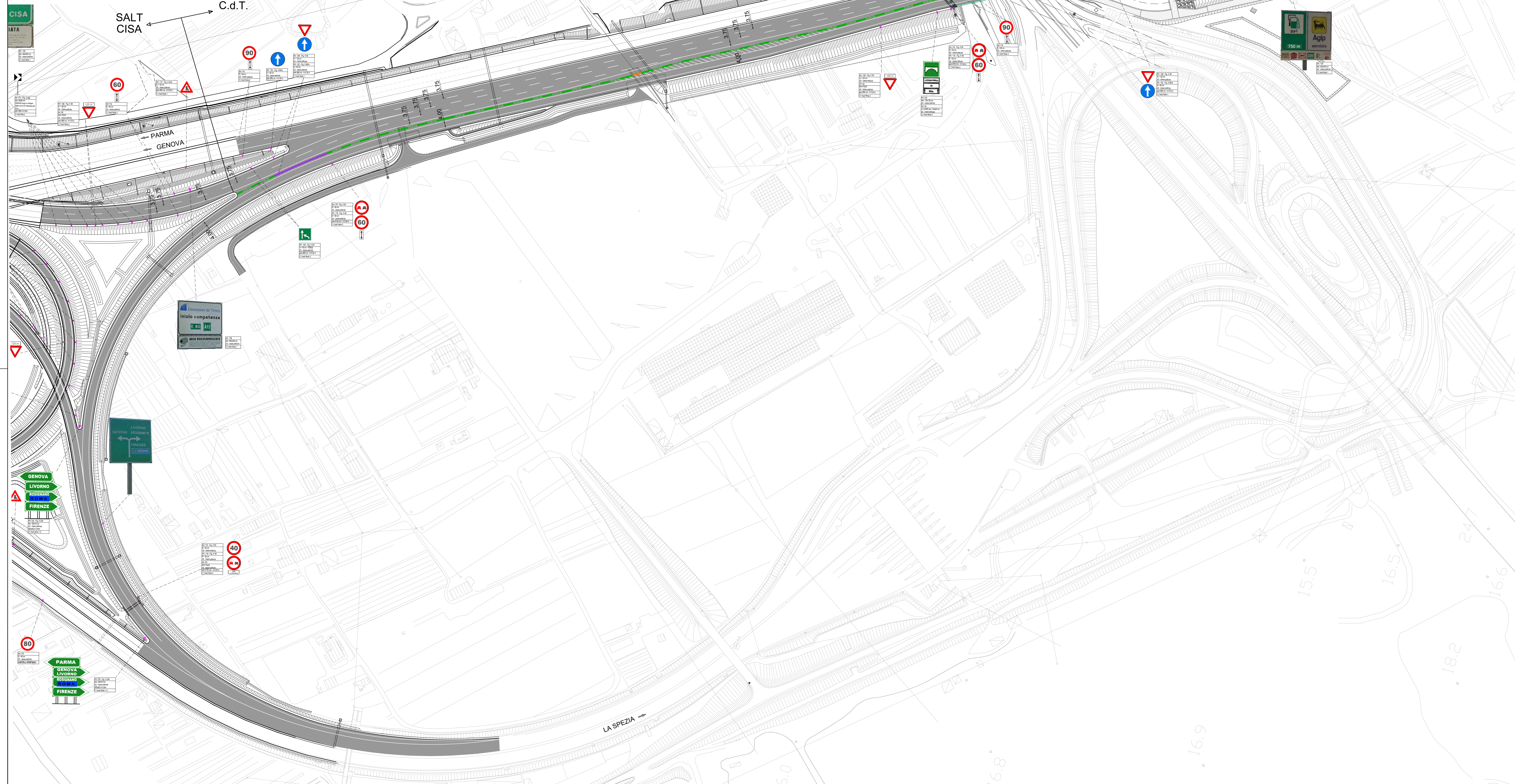
PLANIMETRIA DELLA SEGNALETICA - TAV.2 Scala 1:1000
