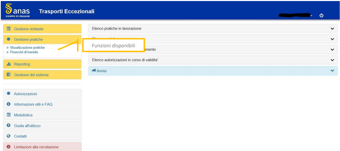
Figura 65 - Gestione pratiche
