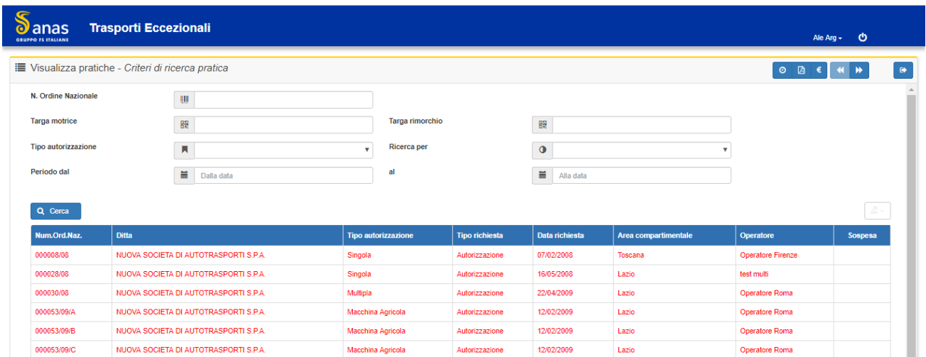
Figura 66 - Visualizzazione pratiche
