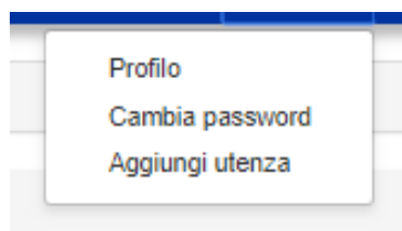
Figura 18 - Gestione Profilo
