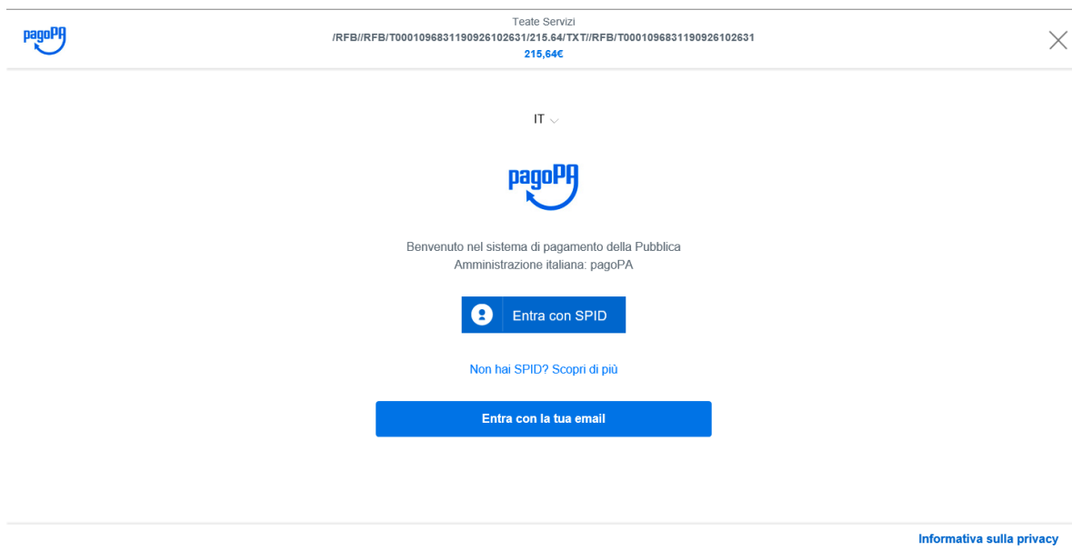
Figura 64 – pago PA
