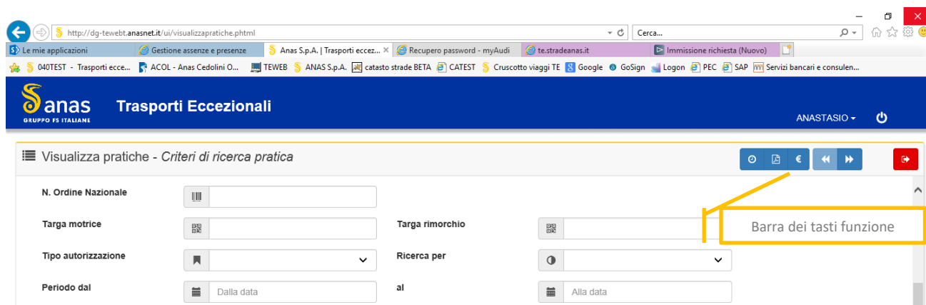
Figura 21 – Tasti funzione
