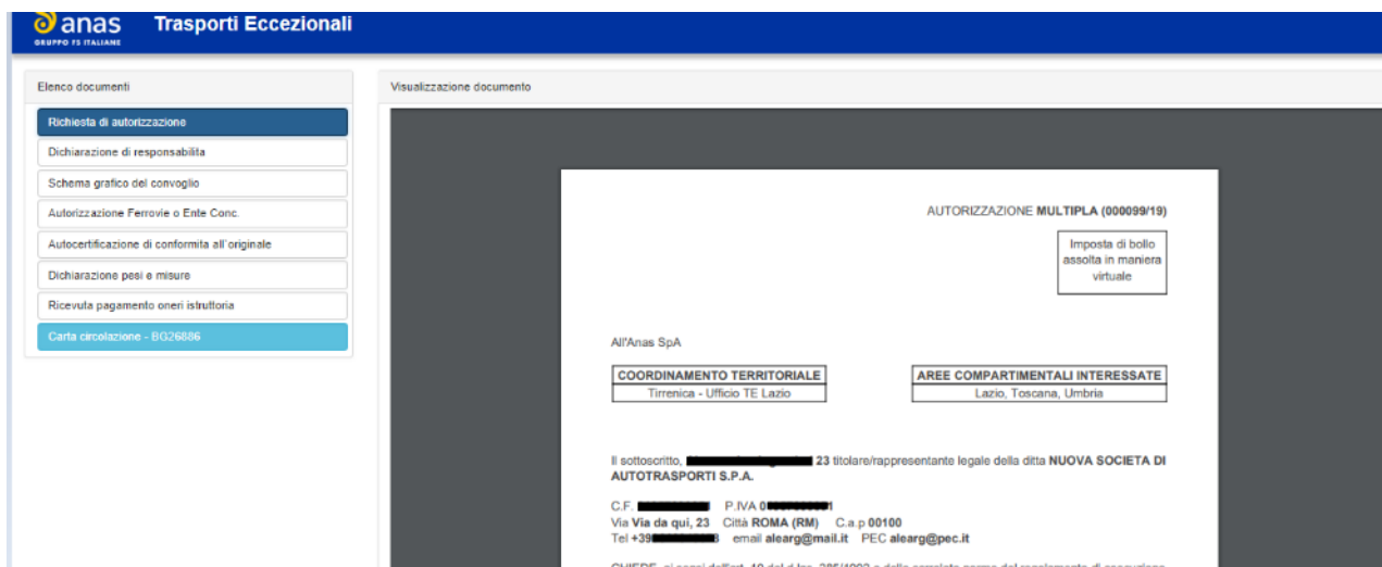
Figura 23 – Visualizza PDF
