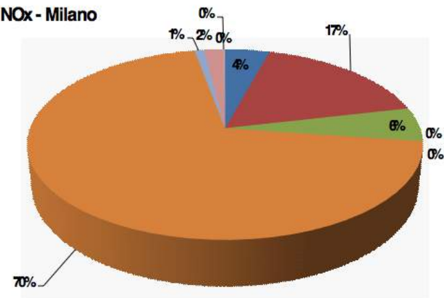
NOx - Milano
