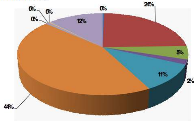
PM10 - Milano
